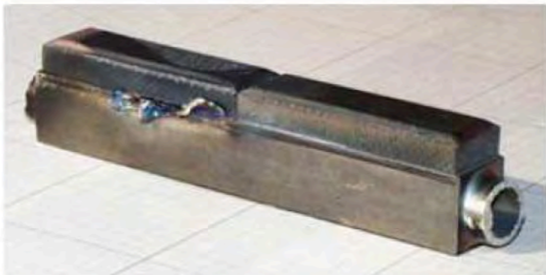
Un élément de première paroi détruit en opération (1999)
